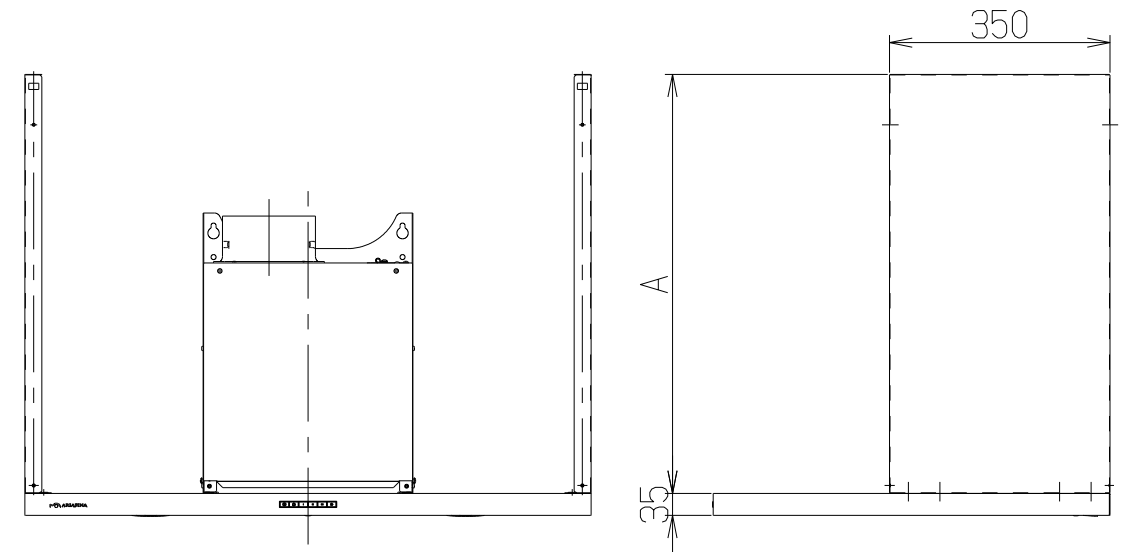
施工例
