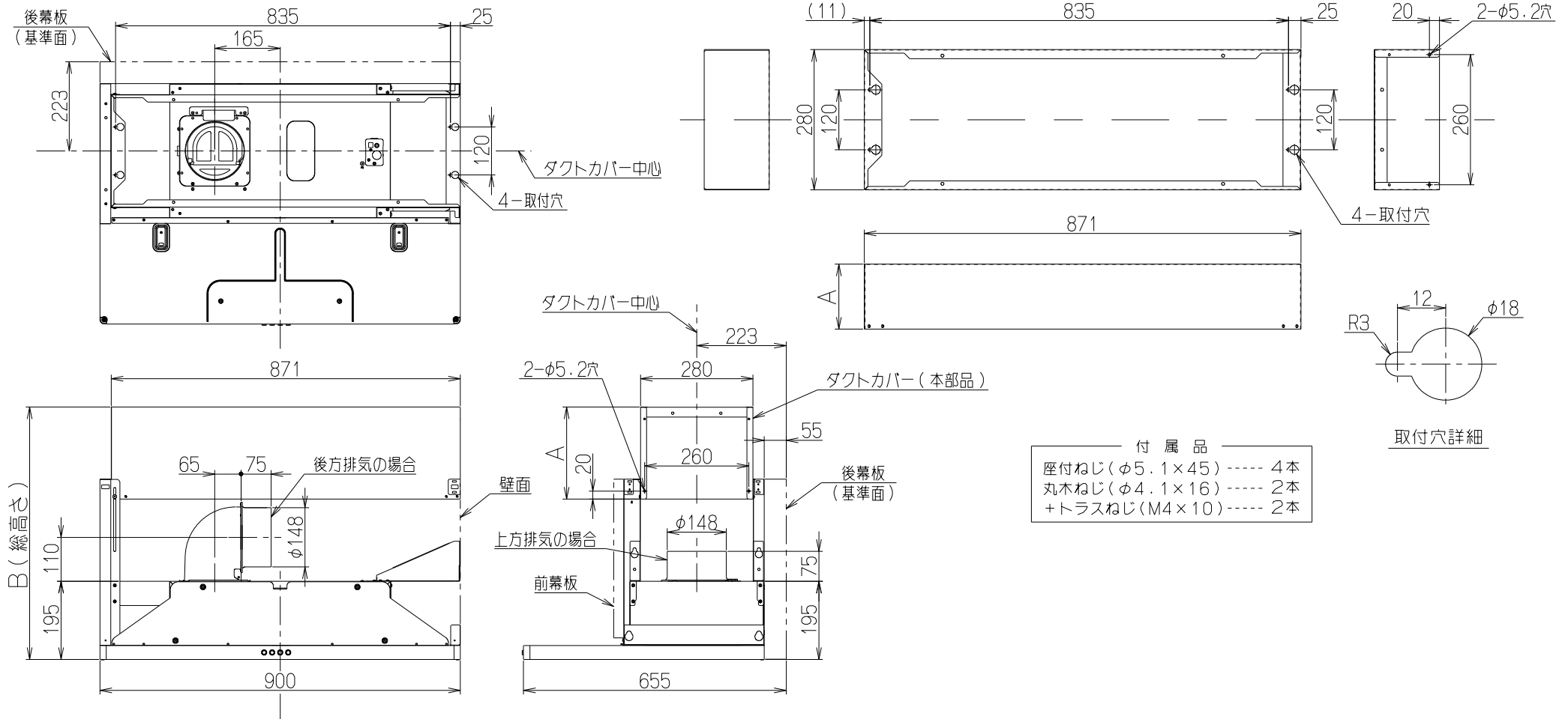
取付例
